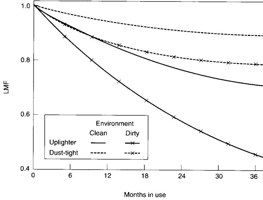
Коефициент на нечистотија на светилките
