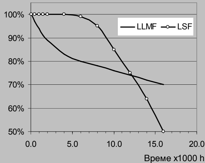
ФС (халофосфати)
